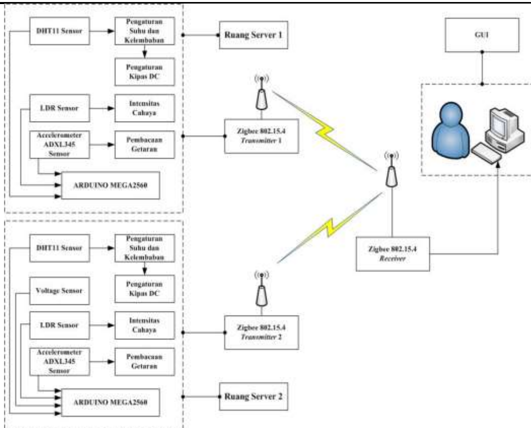
Gambar 2. Diagram Blok Perancangan Perangkat Keras
